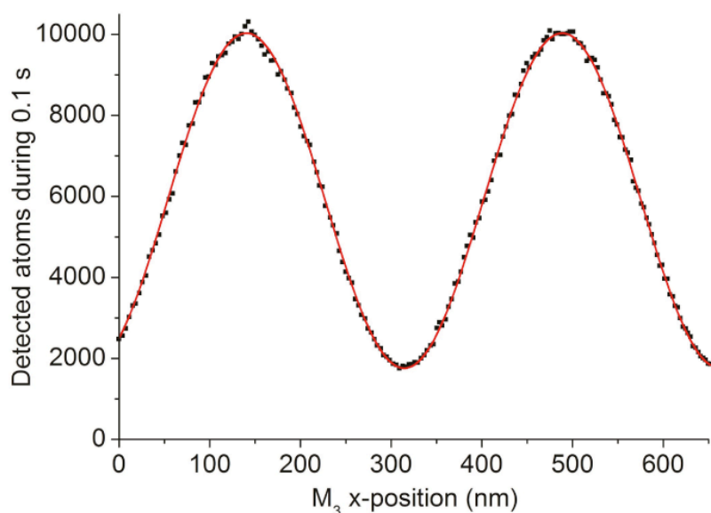
fig. 1 : franges d'interférences enregistrées en l'absence de toute perturbation - © LCAR-IRSAMC
