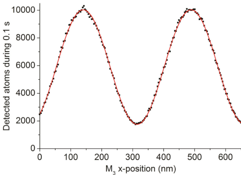
fig. 1 : franges d'interférences enregistrées en l'absence de toute perturbation - © LCAR-IRSAMC
